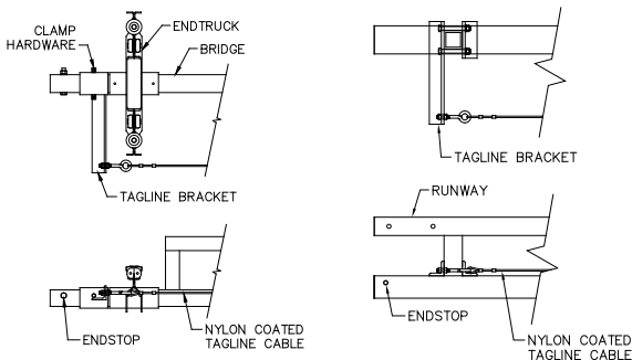
Diagram 9A. Tagline on bridge.
